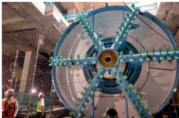
Ảnh 1+2+3. Metro Line 1 (TP HCM) Vận hành máy khoan hầm TBM
